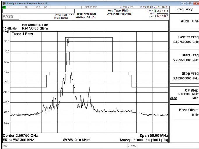
Band 7_QPSK_15M_RB1,74
