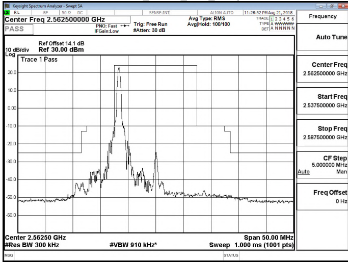
Band 7_QPSK_15M_RB1,74
