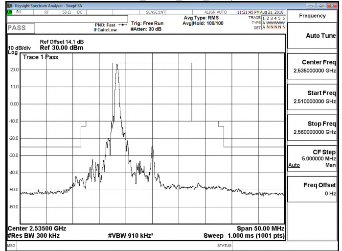
Band 7_QPSK_15M_RB1,74
