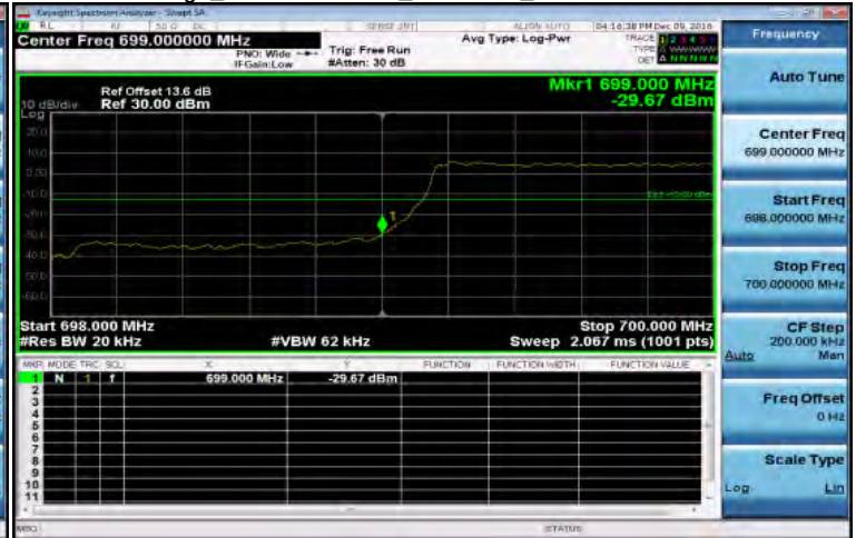
Band Edge_Band12 1.4MHz_QPSK 6 0_LowCH23017-699.7
