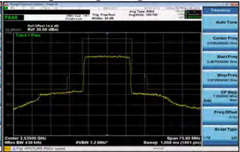
Mask_Band7 20MHz_QPSK 100 0_ MidCH21100-2535
