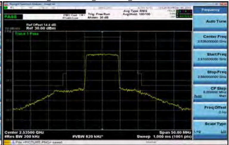
Mask_Band7 10MHz_QPSK 50 0_MidCH21100-25355
