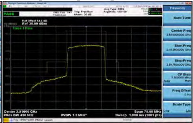
Mask_Band7 20MHz_QPSK 100 0_ LowCH20850-2510
