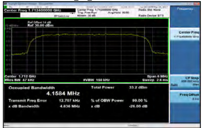
WCDMA_B4_LowCH1312-1712.4
