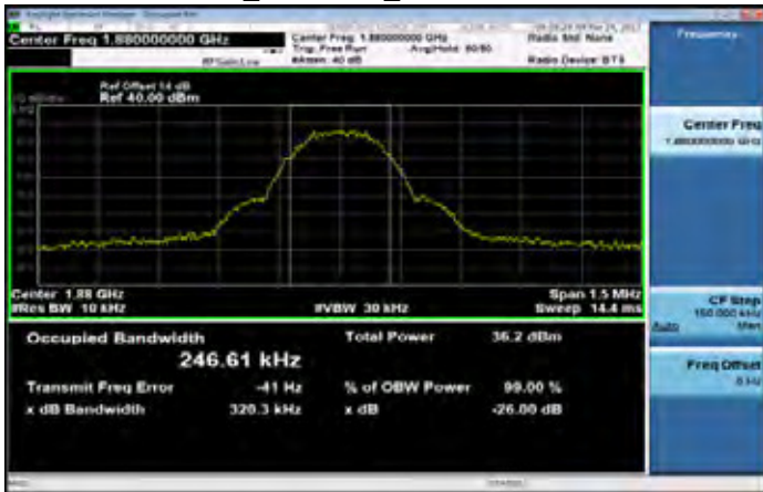
GPRS_1900MHz_MidCH661-1880
