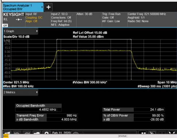
5MHz / QPSK
