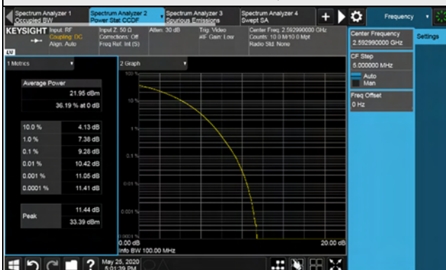
100MHz / 256QAM
