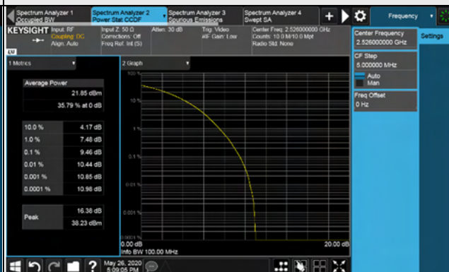
90MHz / 256QAM
