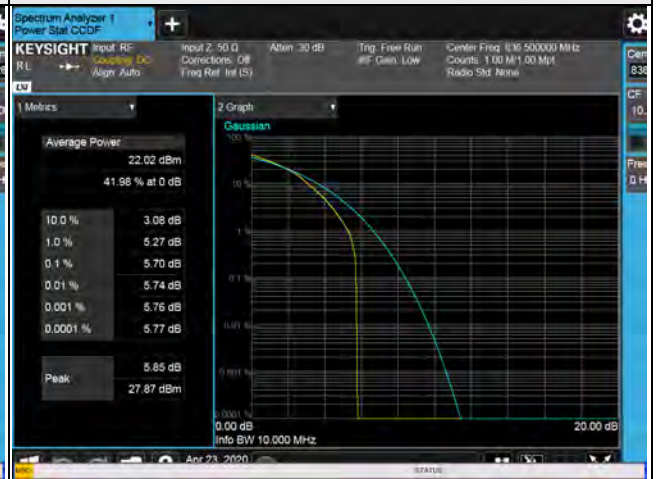
10MHz / 64QAM
