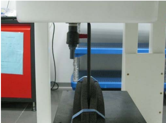
Fig.4 EUT Left Edge to flat phantom
