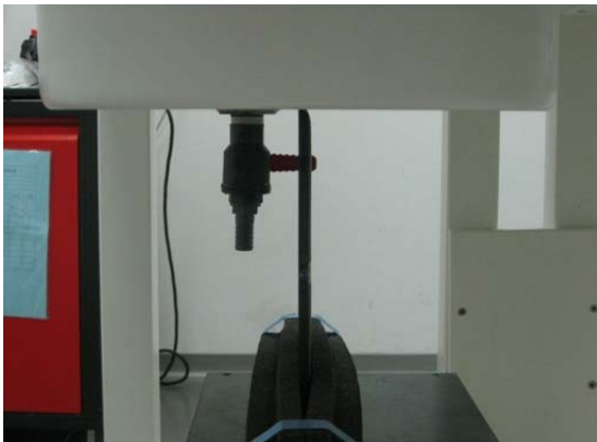
Fig.5 EUT Right Edge to flat phantom
