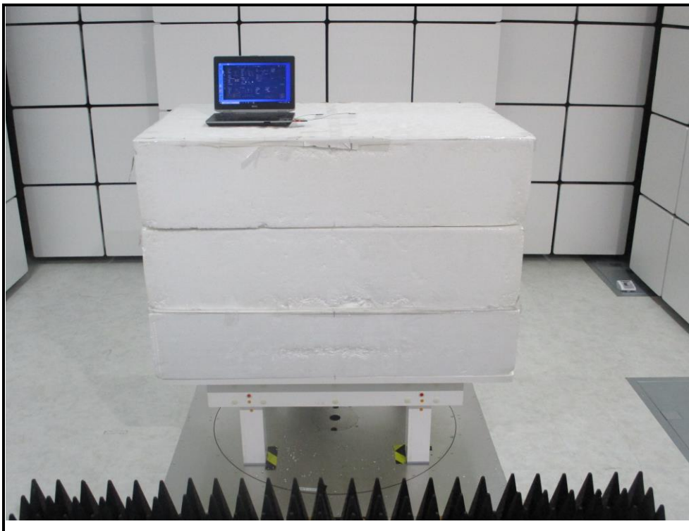
PIFA Antenna 2TX
