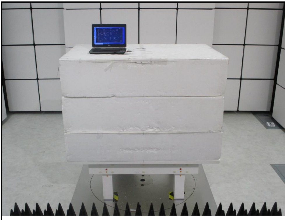
PIFA Antenna 1TX
