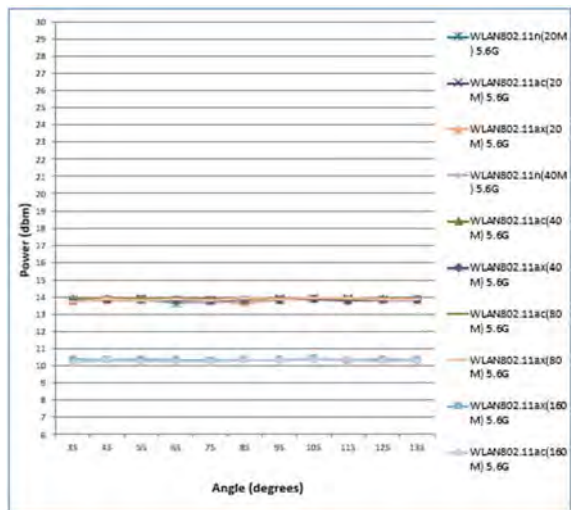
5.6GHz Tx2(MIMO)
