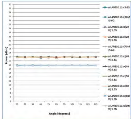
5.6GHz Tx2(SISO)
