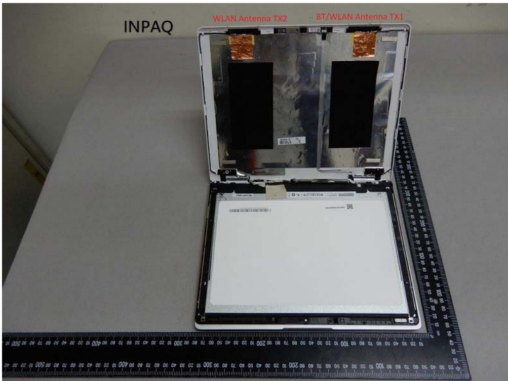
Antenna (Supplier: INPAQ)
