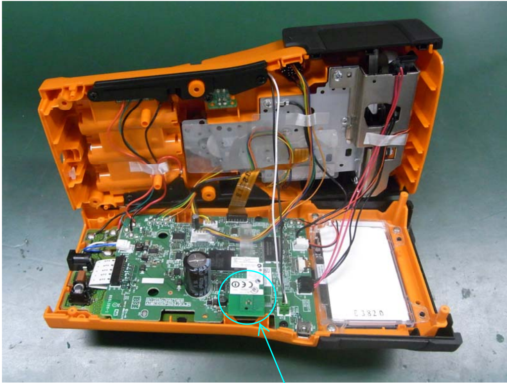
IEEE802.11 b/g/n Module
