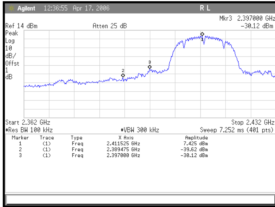
Plot 27. 802.11/g – DSSS Lower Band Edge
