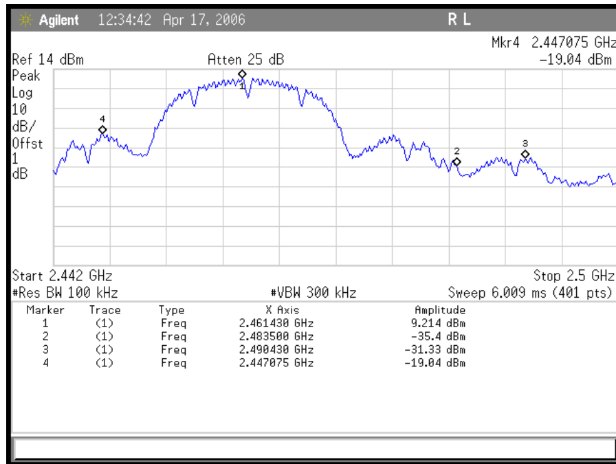
Plot 28. 802.11/g – DSSS Upper Band Edge
