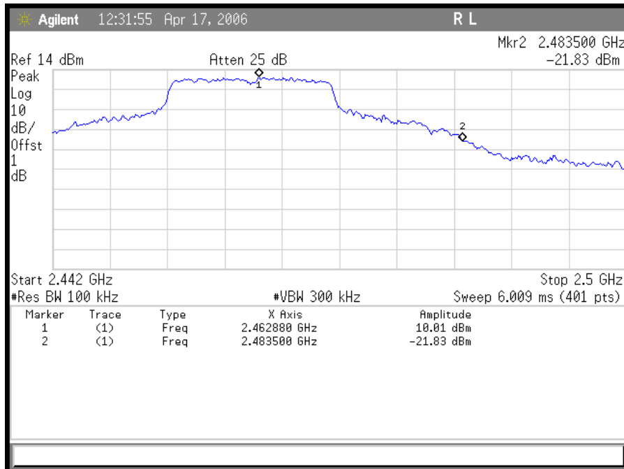
Plot 30. 802.11/g – OFDM Upper Band Edge
