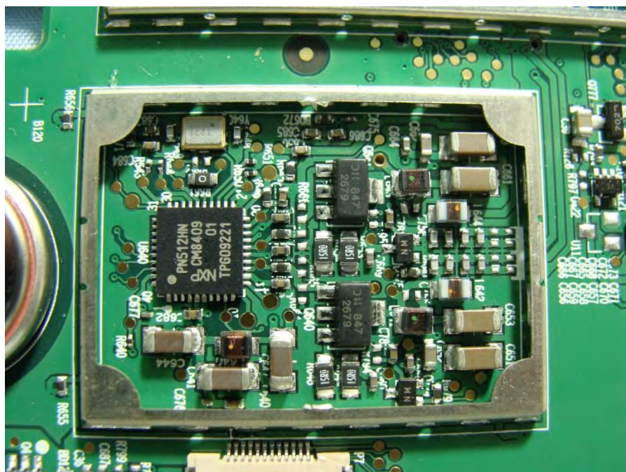
RFID module
