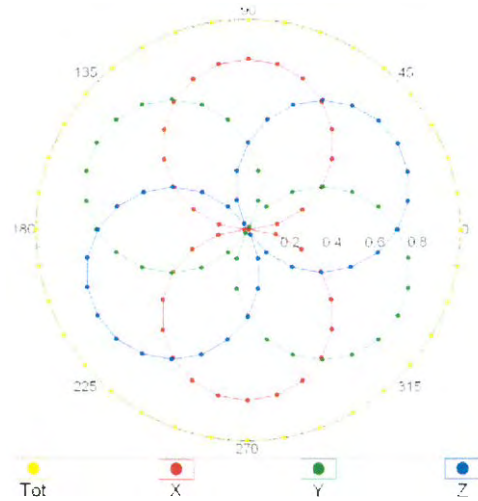
f=1800 MHz,R22
