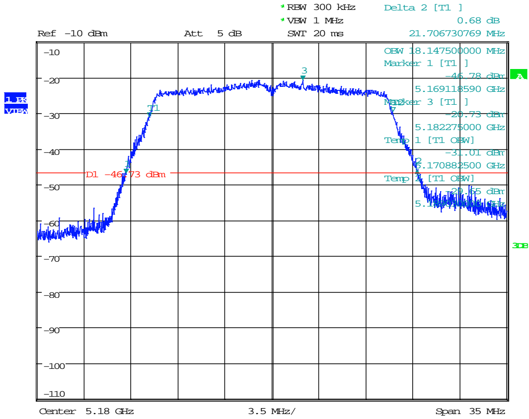
Plot 1. 4 802.11n 20MHz, 5180MHz
