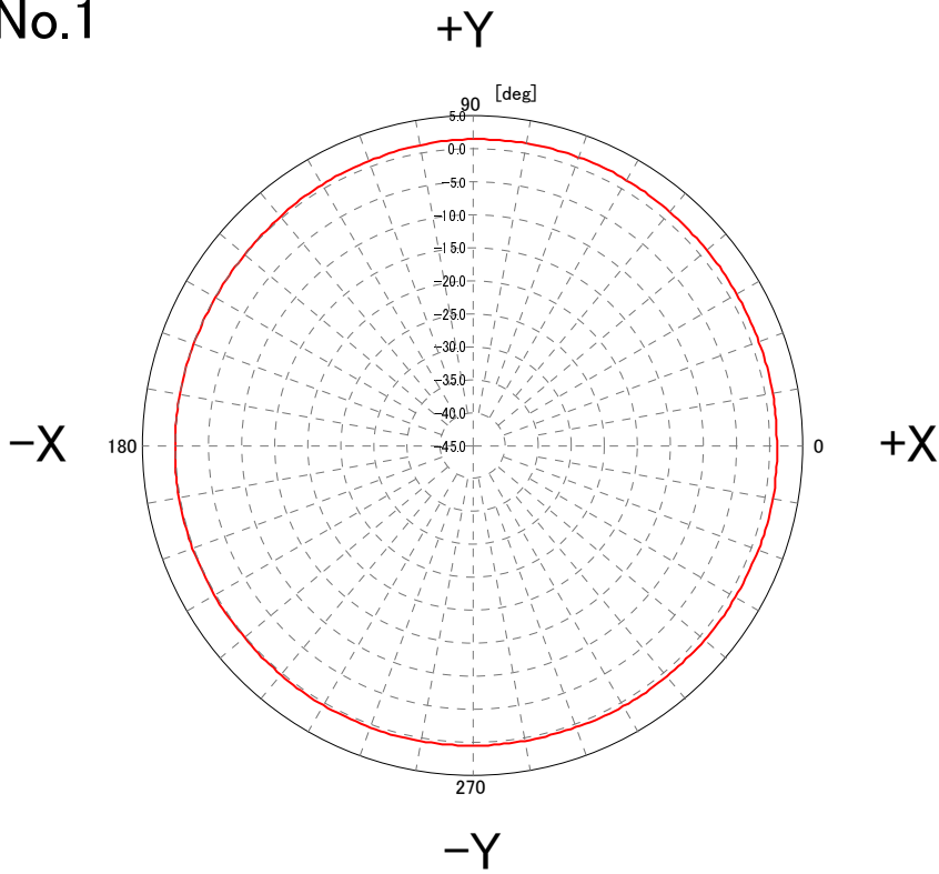
2500MHz / X-Y面 X-Y Face
