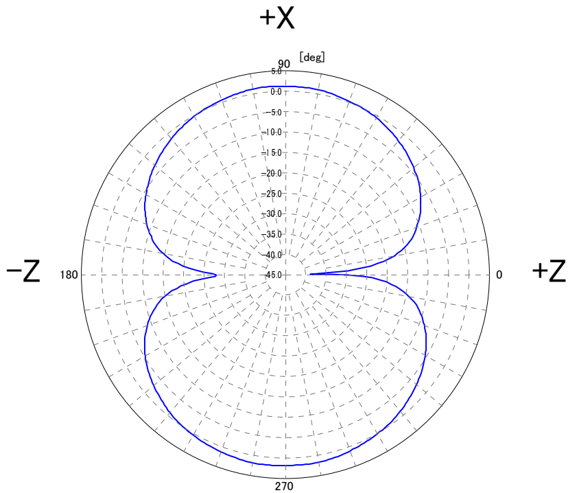
-X 2450MHz / Z-X面 Z-X Face
