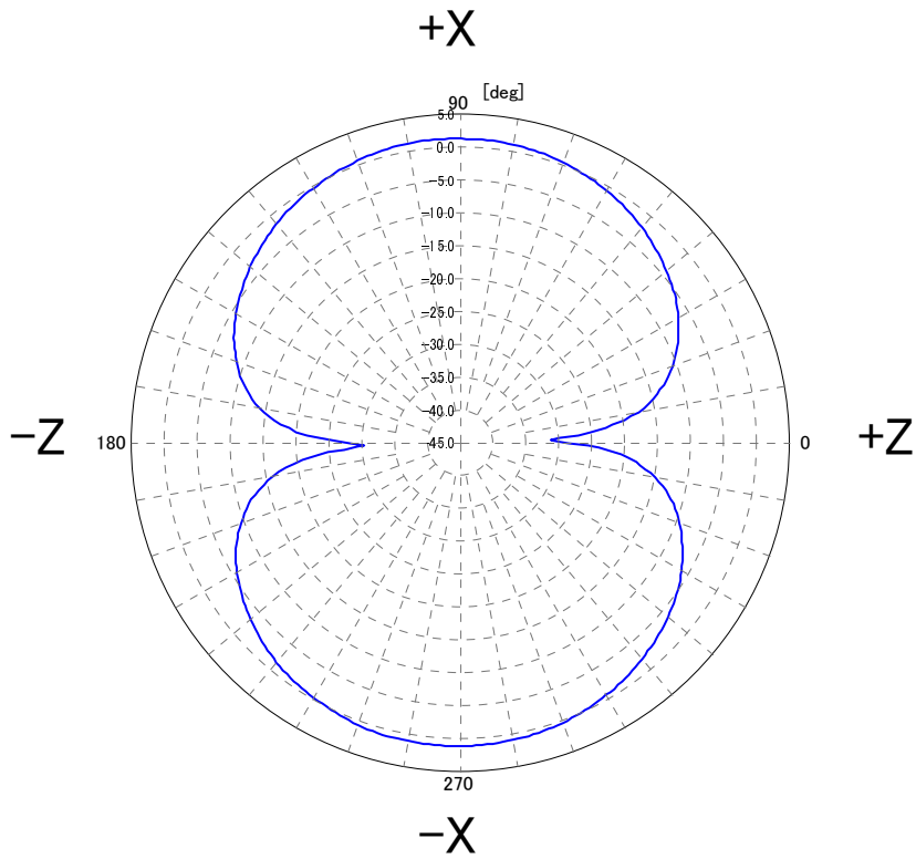
2500MHz / Z-X面 Z-X Face
