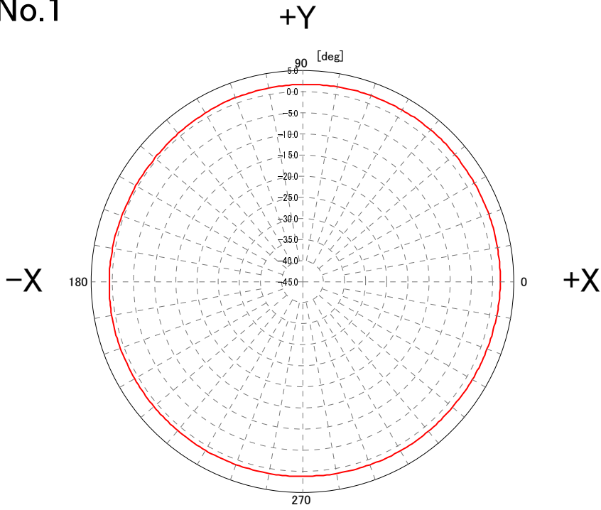
-Y 2450MHz / X-Y面 X-Y Face
