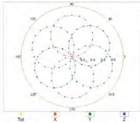
f=1800 MHz,R22
