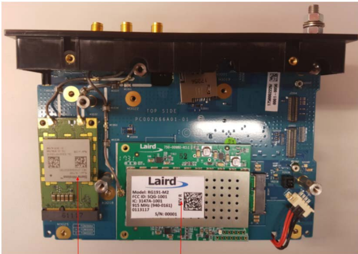
LTE Module
