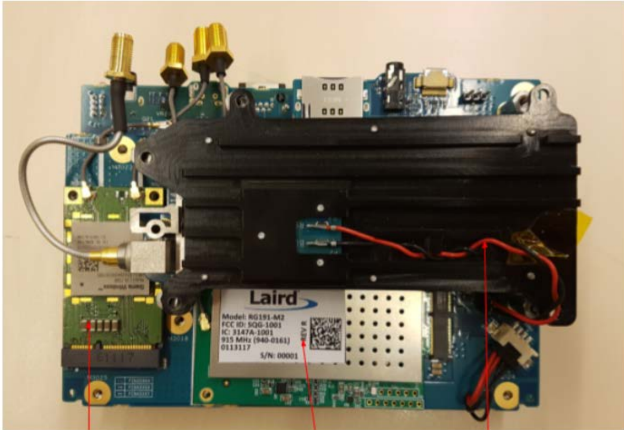
LTE Module
