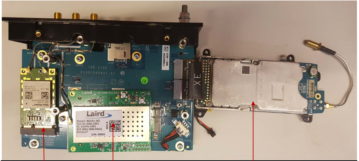
LTE Module
