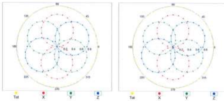
f=1800 MHz,R22
