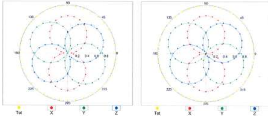
f=1800 MHz,R22
