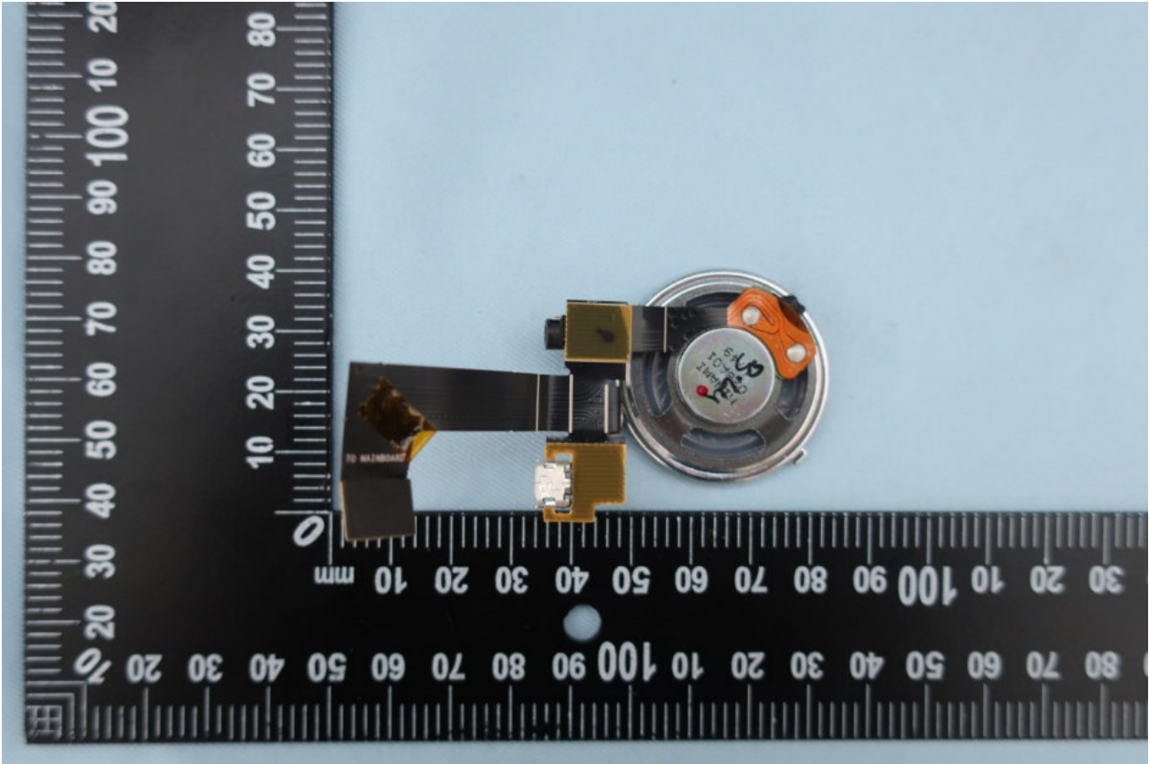
<Speaker_mic_USB_audiojack FPCA bottom side>
