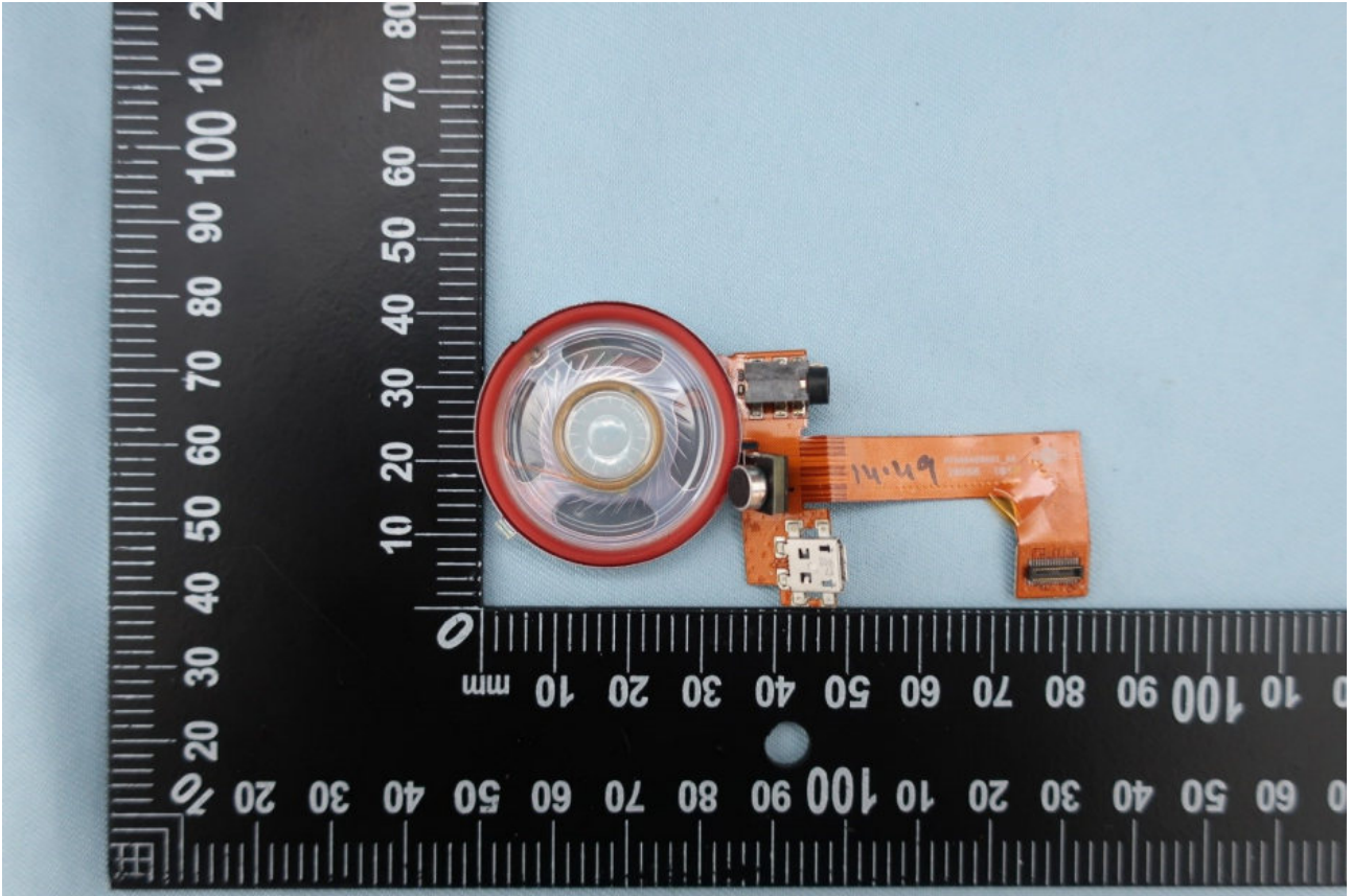
<Speaker_mic_USB_audiojack FPCA top side>
