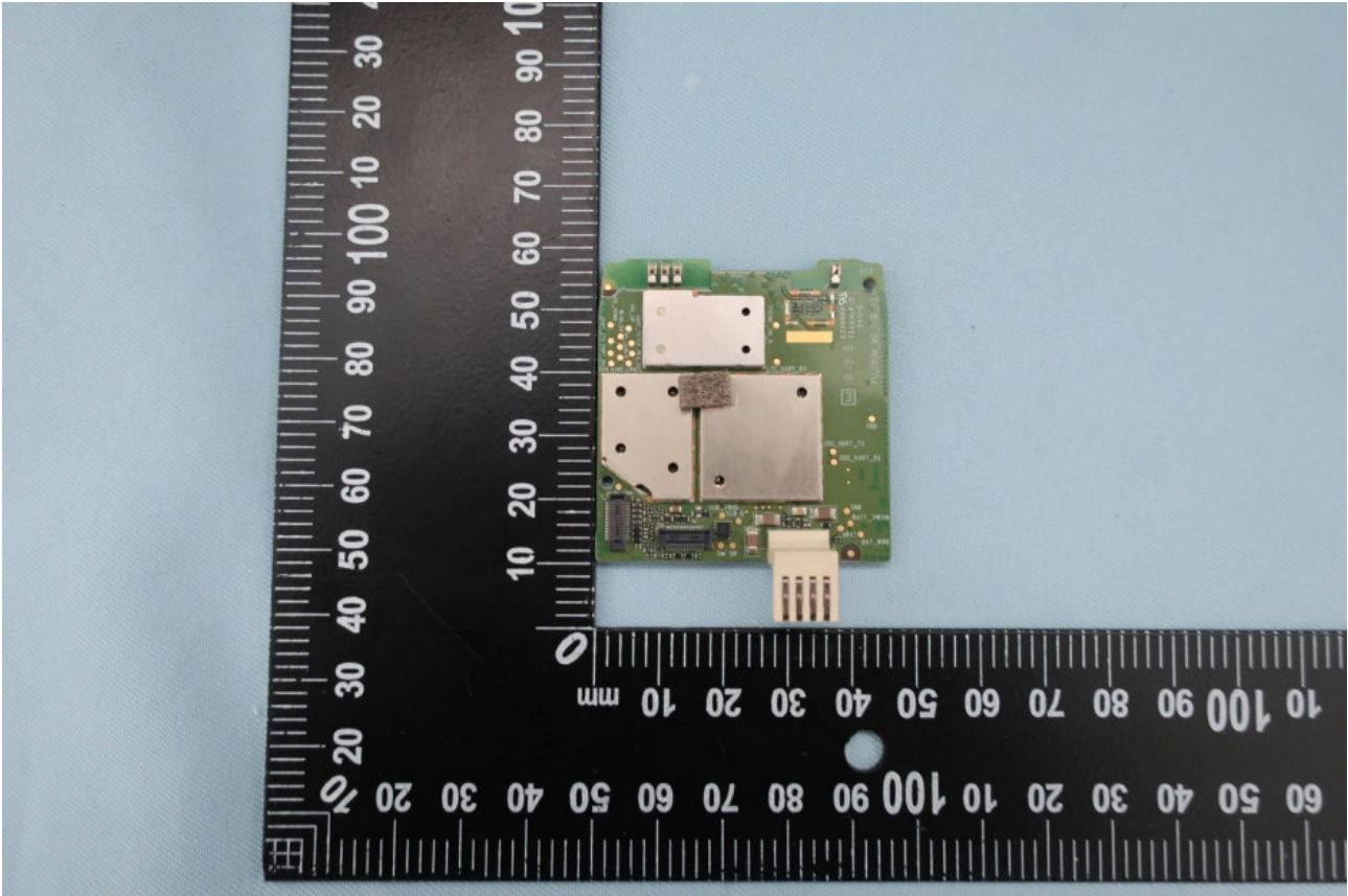
<Main PCBA top side>
