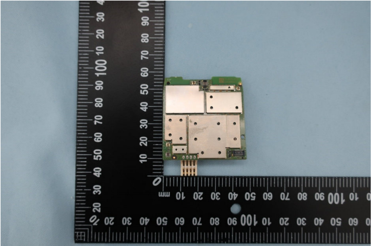
<Main PCBA bottom side>
