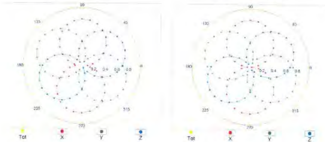
f=1800 MHz,R22
