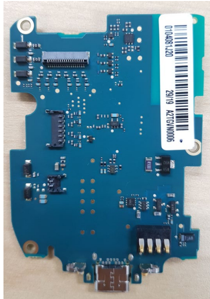
PCB Bottom
