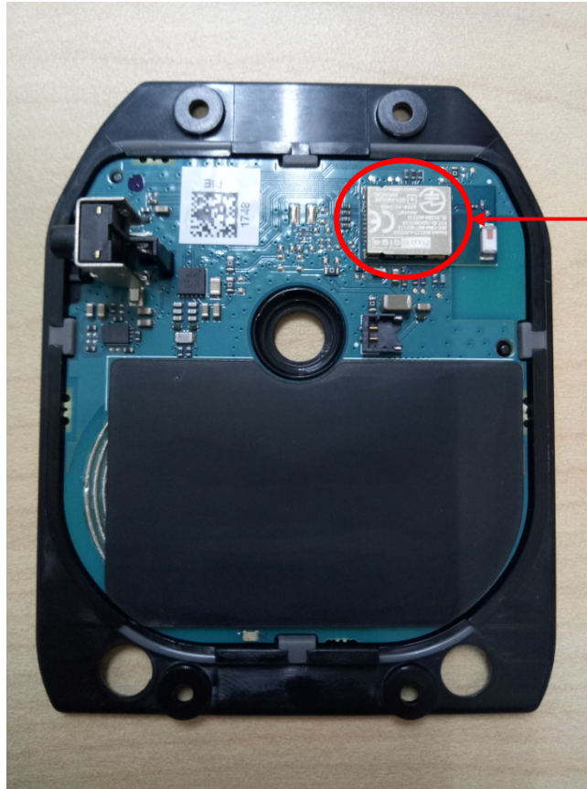
PCB Top
