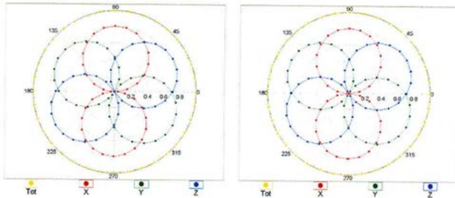
f=1800 MHz,R22
