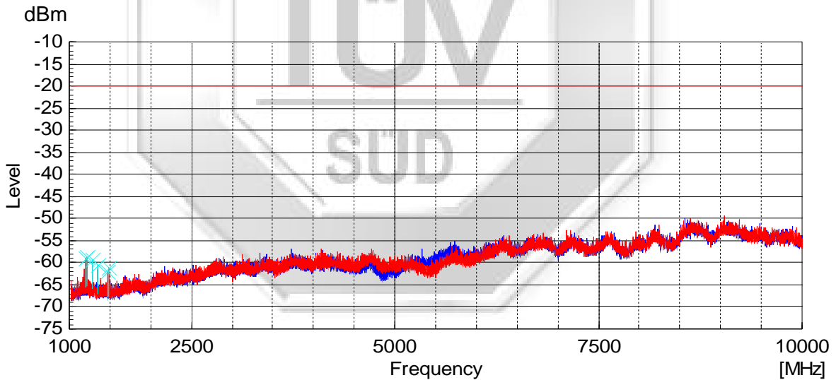
158.55MHz (Digital) 1GHz – 10GHz
