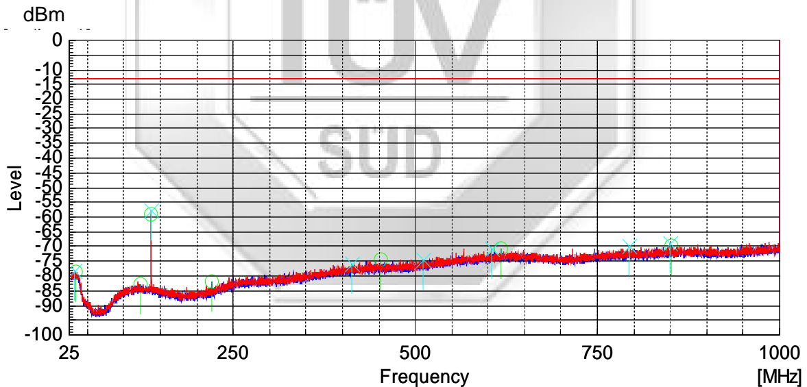
138.0125MHz (Analog) 25MHz – 1GHz
