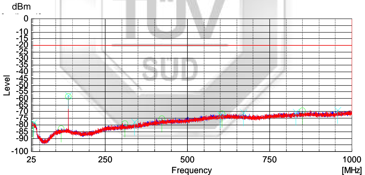
138.0125MHz (Digital) 25MHz – 1GHz
