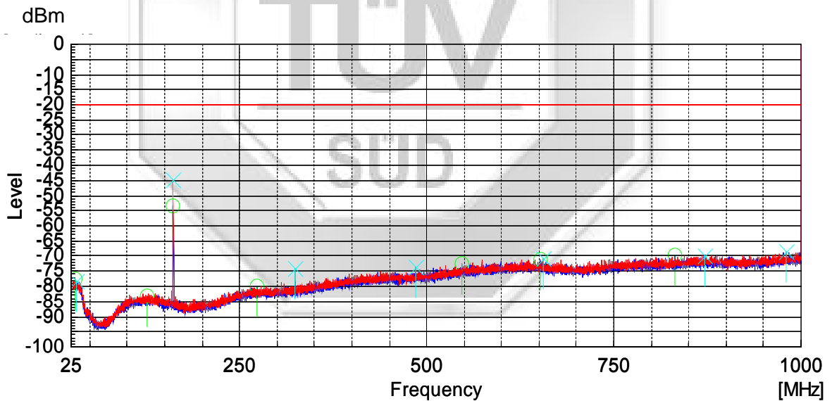
161.7MHz (Digital) 25MHz – 1GHz
