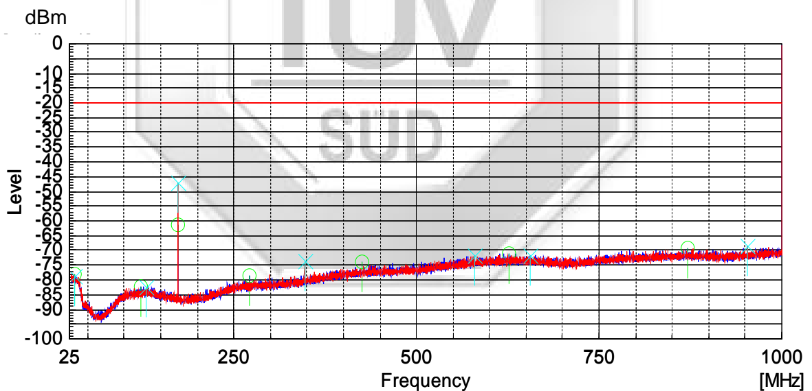
173.3875MHz (Digital) 25MHz – 1GHz
