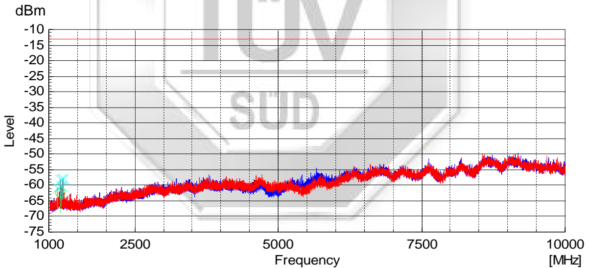
138.0125MHz (Analog) 1GHz – 10GHz
