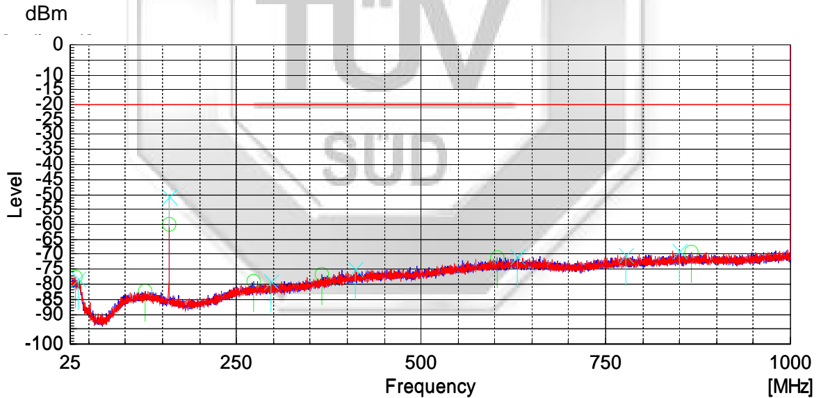
158.55MHz (Digital) 25MHz - 1GHz
