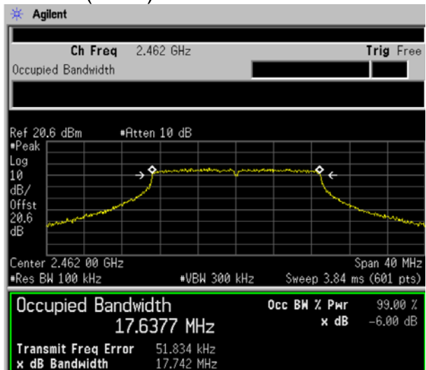
802.11n(HT20) 2462MHz
