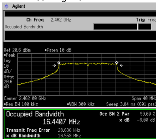
802.11g 2462MHz
