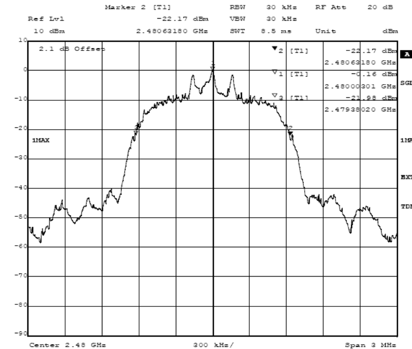
Title: 20dB Bandwidth Comment A: CH T: 2480 MHz; 20dB bandwidth (kHz):1251.6
