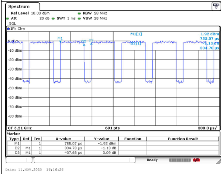
802.11ac_VHT80
