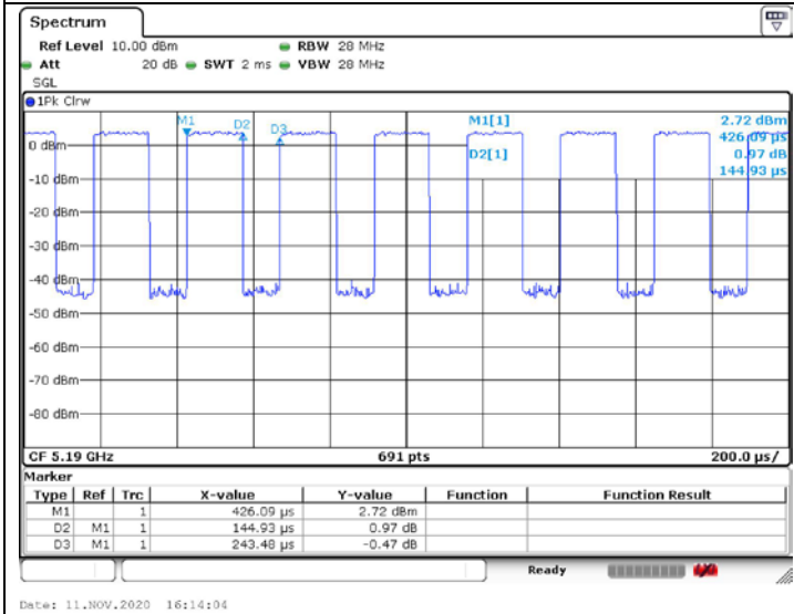
802.11n_HT40
