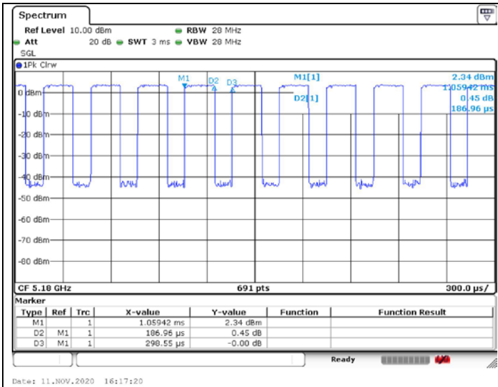
802.11n_HT20
