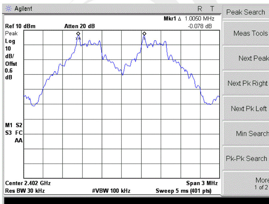
CH00 -1Mbps
