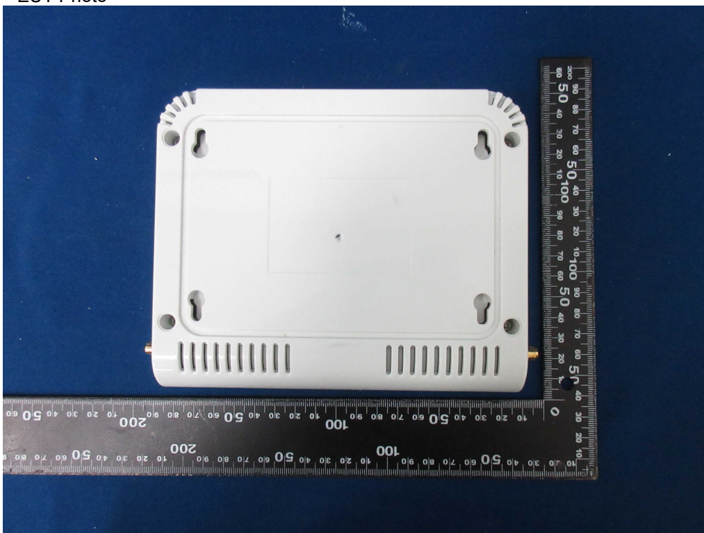
(2) EUT Photo
