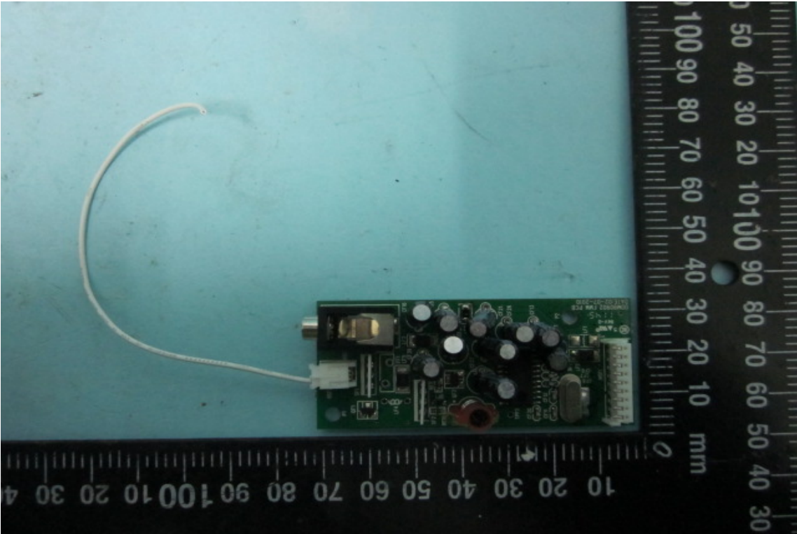
14. RF Module
