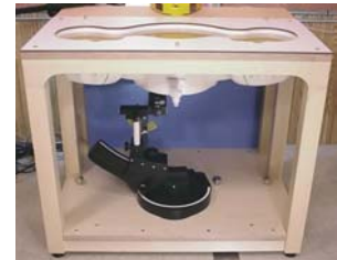
SAM Phantom
