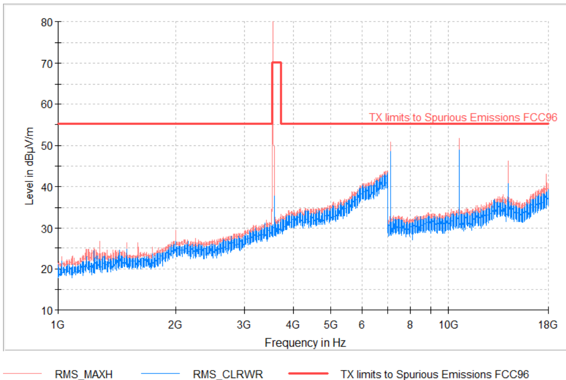
RF_FCC_Part96_E Field_1GHz_18GHz
