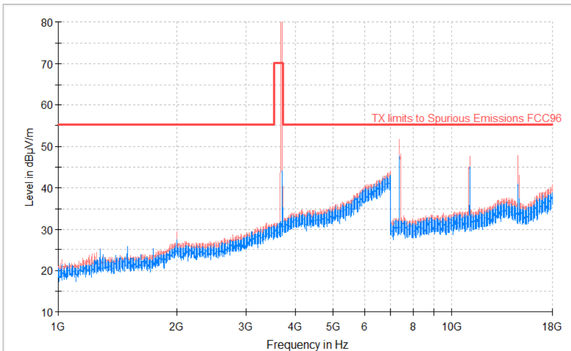
RF_FCC_Part96_E Field_1GHz_18GHz
