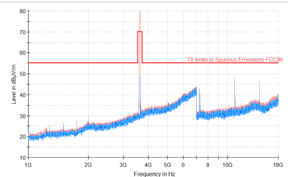
RF_FCC_Part96_E Field_1GHz_18GHz
