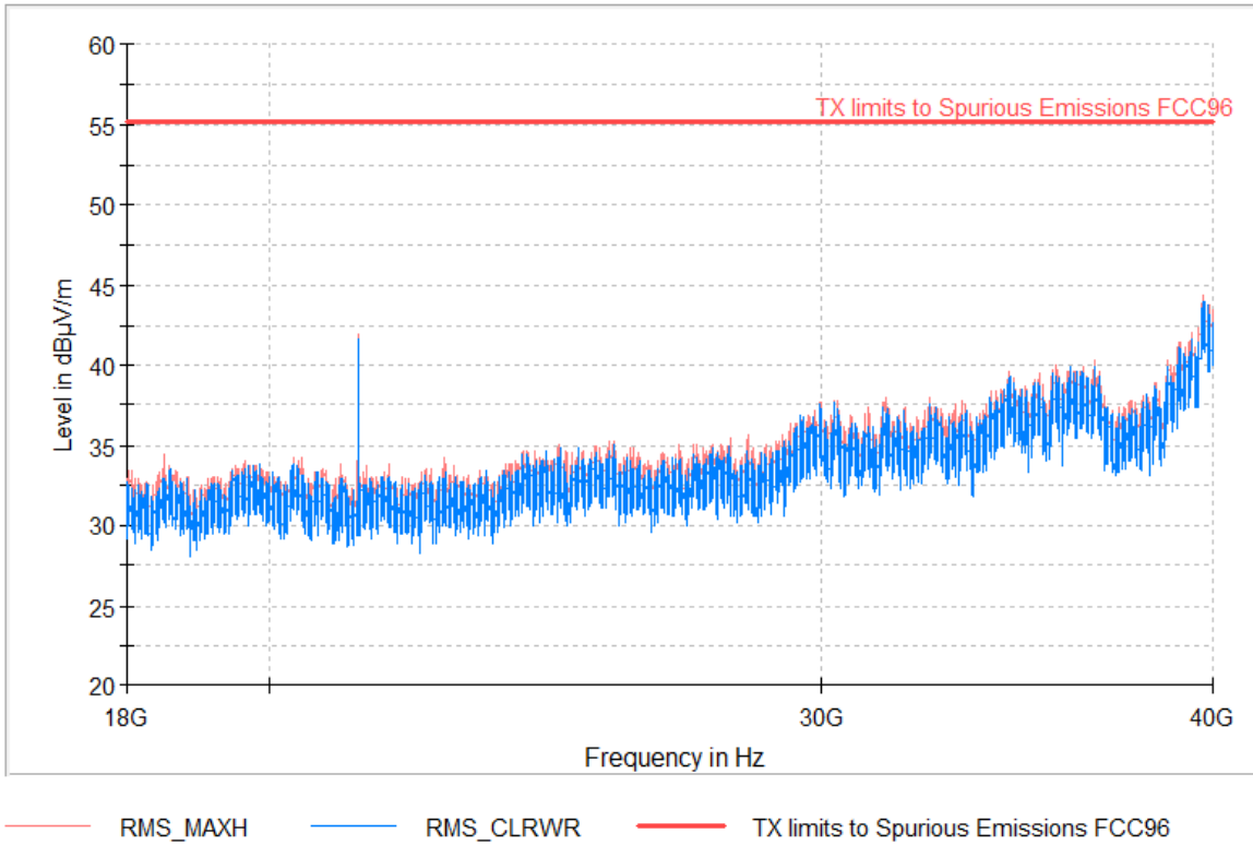
RF_FCC_Part96_E Field_18GHz_40GHz
