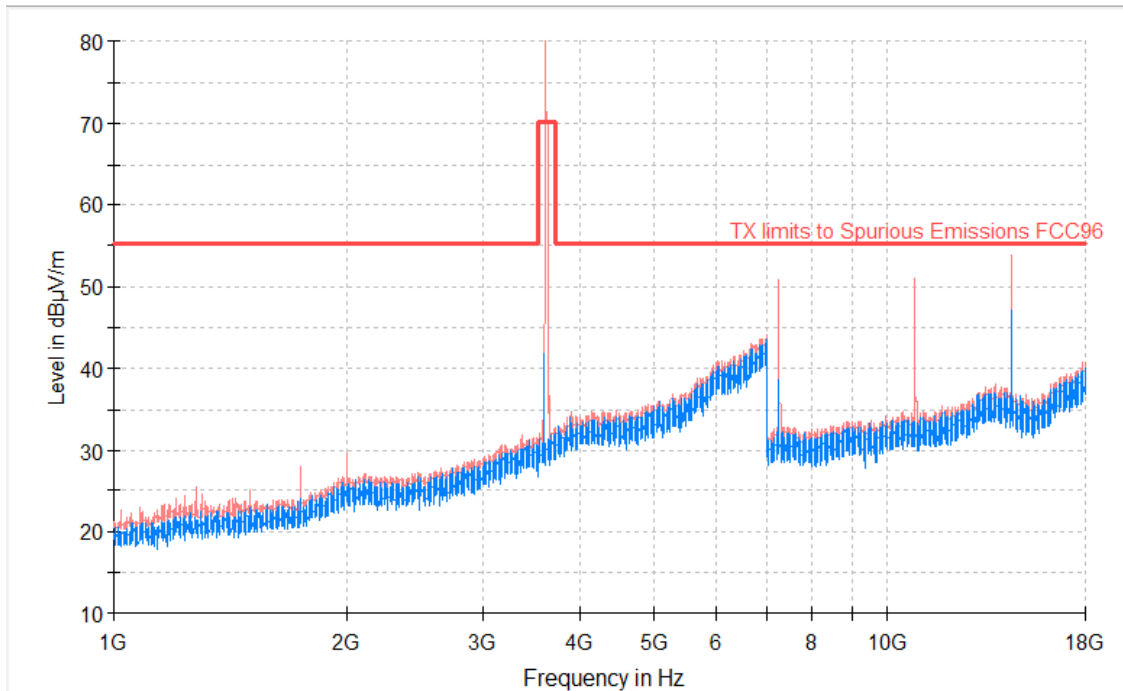
RF_FCC_Part96_E Field_1GHz_18GHz
