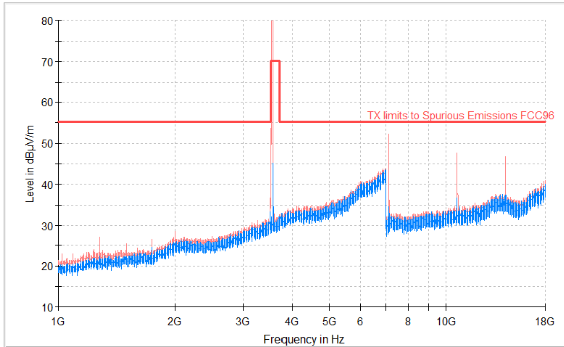
RF_FCC_Part96_E Field_1GHz_18GHz
