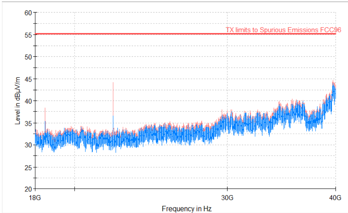
RF_FCC_Part96_E Field_18GHz_40GHz
