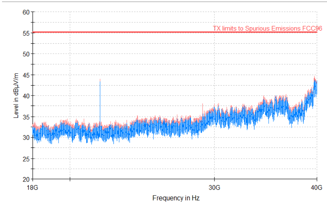
RF_FCC_Part96_E Field_18GHz_40GHz
