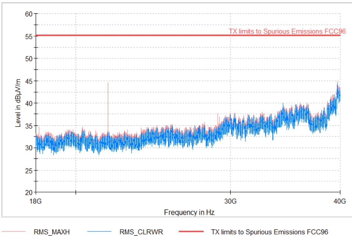
RF_FCC_Part96_E Field_18GHz_40GHz
