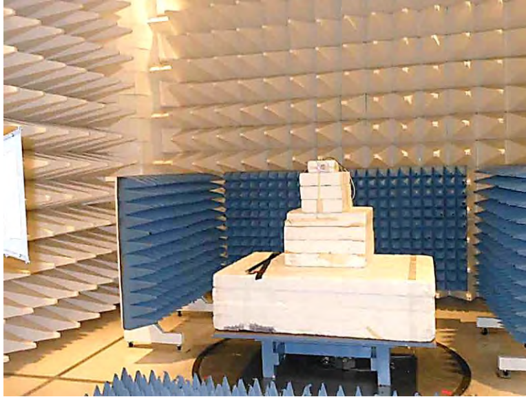
Configuration 1, 1 – 12GHz
