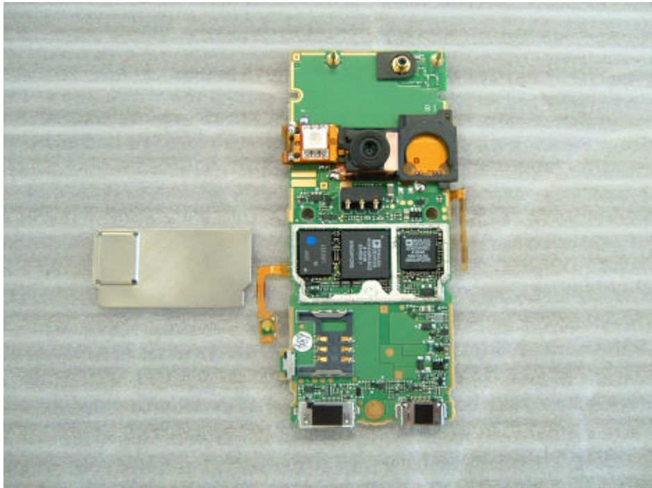
Middle Layer Side B
