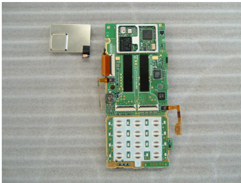
Middle Layer Side A
