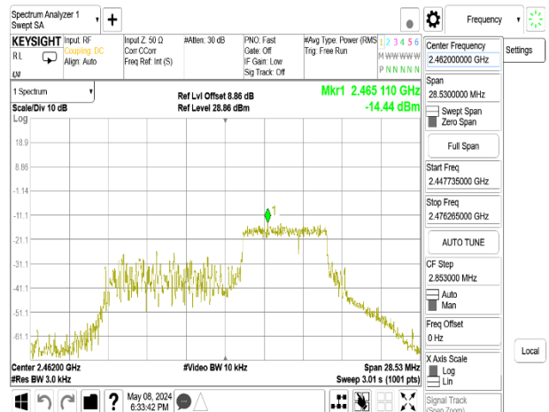
802.11be_20MHz_Chain1_2462MHz_RU106_54
