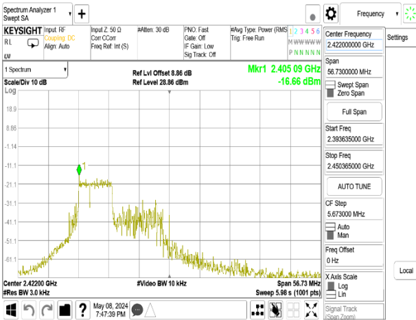
802.11be_40MHz_Chain1_2422MHz_RU242_61
