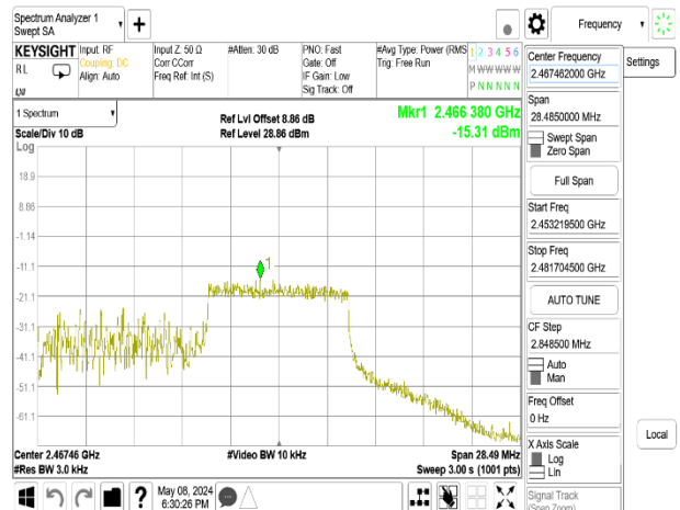
802.11be_20MHz_Chain0_2462MHz_RU26_8
