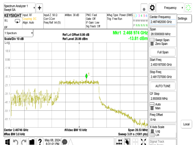
802.11be_20MHz_Chain1_2462MHz_RU106_54
