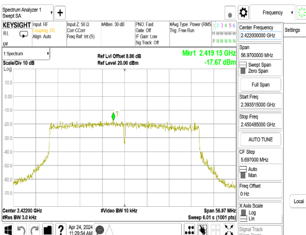
802.11be_40MHz_Chain0_2422MHz
