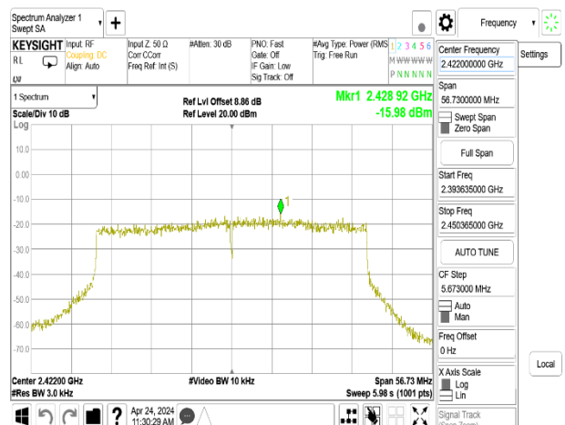
802.11be_40MHz_Chain1_2422MHz
