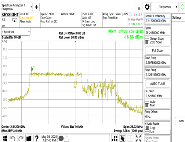
802.11be_20MHz_Chain1_2412MHz_106+26_MRU1
