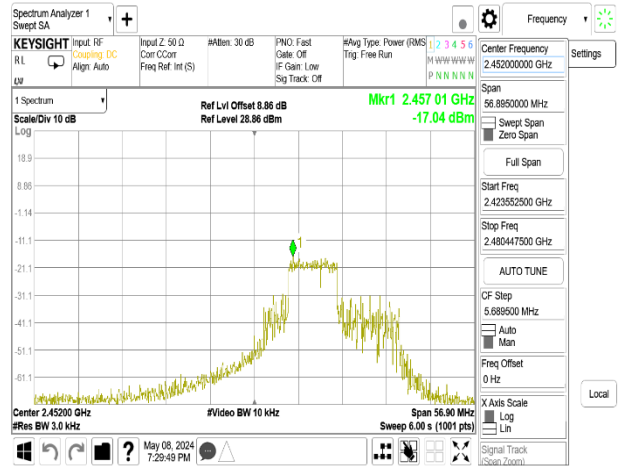
802.11be_40MHz_Chain0_2452MHz_RU242_62
