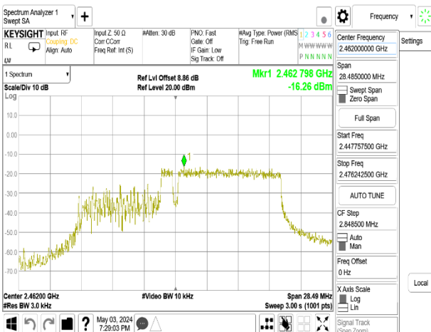
802.11be_20MHz_Chain0_2462MHz_106+26_MRU2
