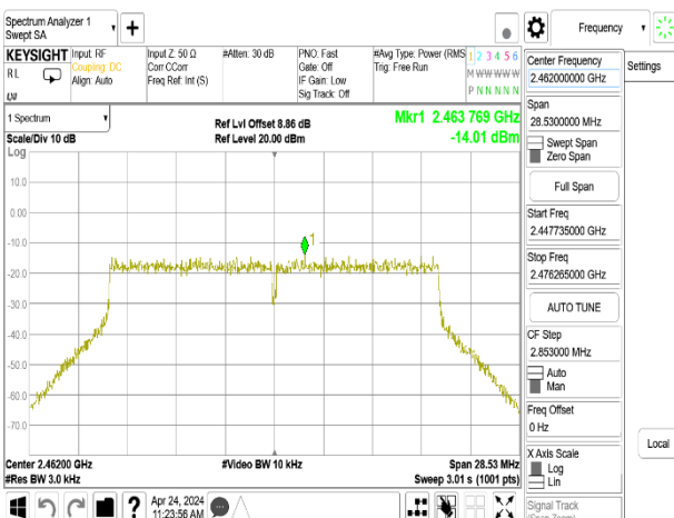
802.11be_20MHz_Chain1_2462MHz
