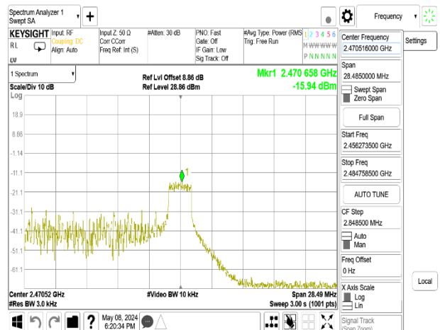
802.11be_20MHz_Chain0_2462MHz_RU26_8
