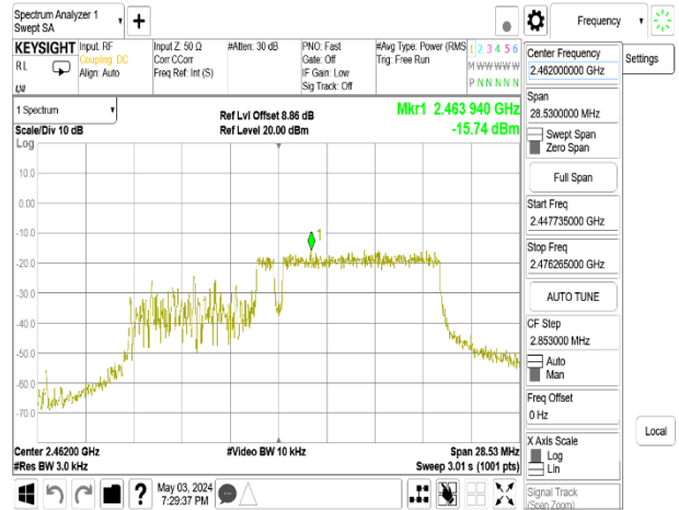
802.11be_20MHz_Chain1_2462MHz_52+26_MRU3
