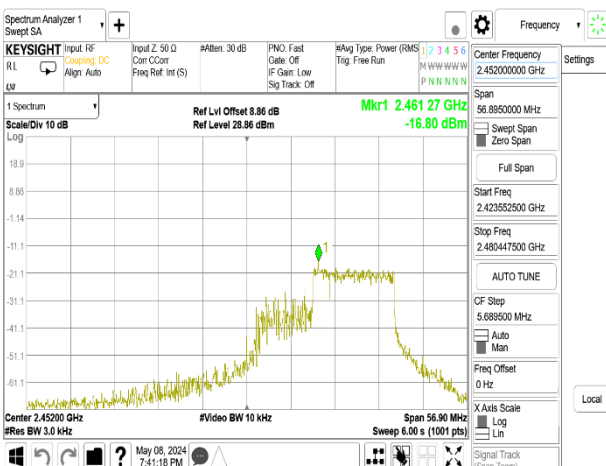
802.11be_40MHz_Chain0_2452MHz_106+26_MRU4
