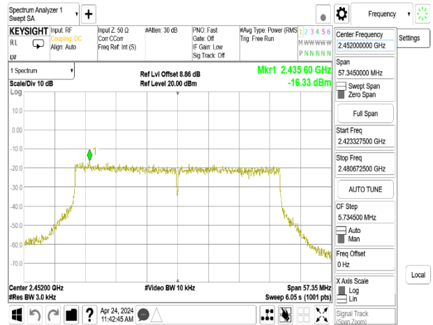
802.11be_40MHz_Chain1_2452MHz_106+26_MRU4
