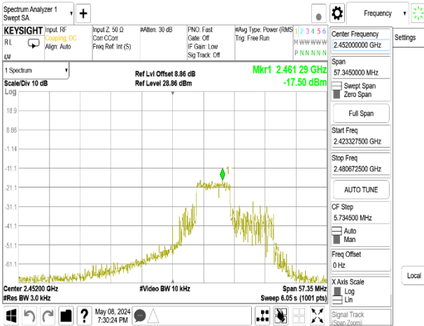
802.11be_40MHz_Chain1_2452MHz_RU242_62
