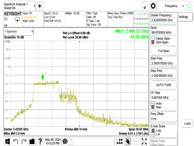
802.11be_40MHz_Chain0_2422MHz_52+26_MRU1
