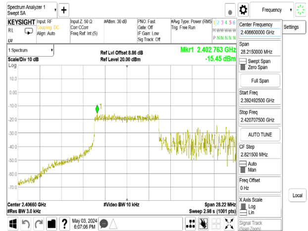
802.11be_20MHz_Chain1_2412MHz_RU26_0
