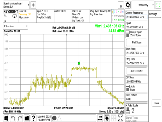
802.11be_20MHz_Chain0_2462MHz_RU106_54
