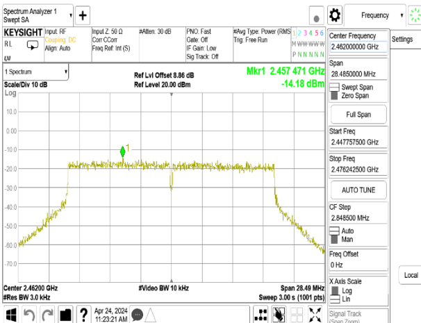
802.11be_20MHz_Chain0_2462MHz_106+26_MRU2
