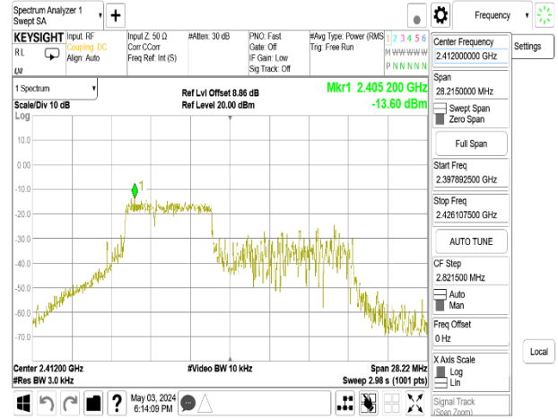
802.11be_20MHz_Chain1_2412MHz_RU106_53
