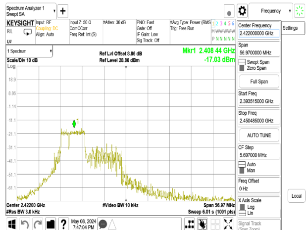
802.11be_40MHz_Chain0_2422MHz_RU242_61
