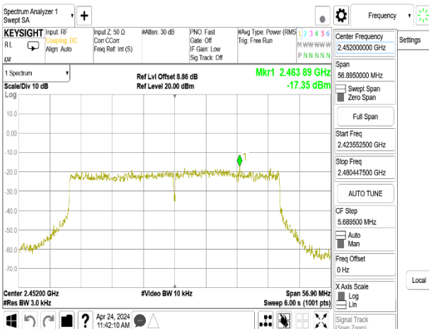
802.11be_40MHz_Chain0_2452MHz_106+26_MRU4
