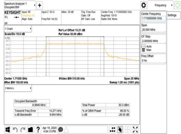
Band4_10MHz_QPSK_RB50_0_CH20175
