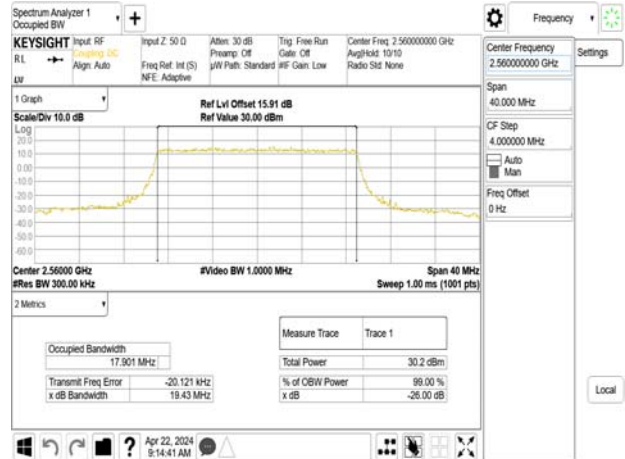
Band7_20MHz_QPSK_RB100_0_CH21350
