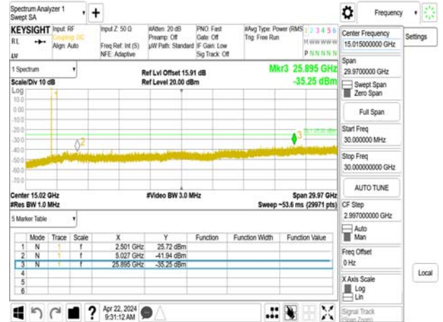
Band7_20MHz_QPSK_RB1_0_CH21100
