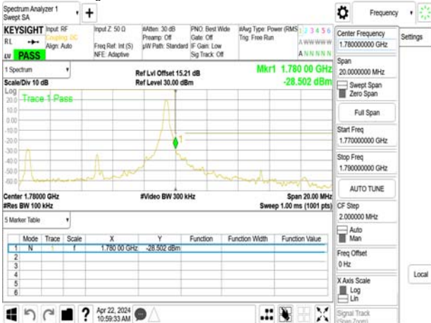
Band Edge_Band66_10MHz_QPSK_RB1_49_CH132622
