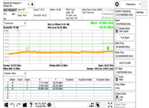
Band4_20MHz_QPSK_RB1_0_CH20175
