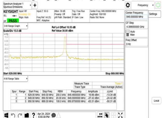
Band5_20MHz_CP_OFDM_SCS15kHz_QPSK_RB1_105_CH167800
