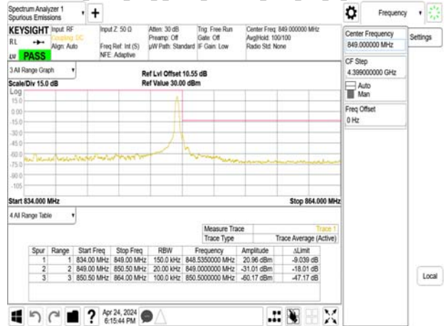
Band5_15MHz_DFT_s_OFDM_SCS15kHz_BPSK_RB1_78_CH168300
