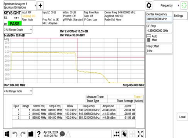
Band5_15MHz_CP_OFDM_SCS15kHz_QPSK_RB79_0_CH168300
