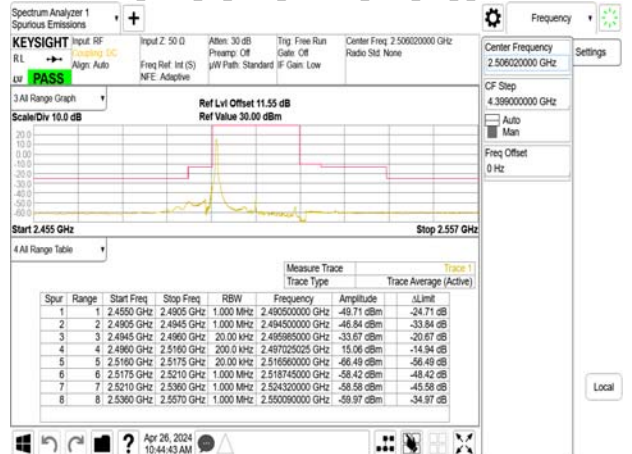
Band41_20MHz_CP_OFDM_SCS30kHz_QPSK_RB1_0_CH501204
