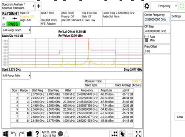
Band41_60MHz_CP_OFDM_SCS30kHz_QPSK_RB1_161_CH505200
