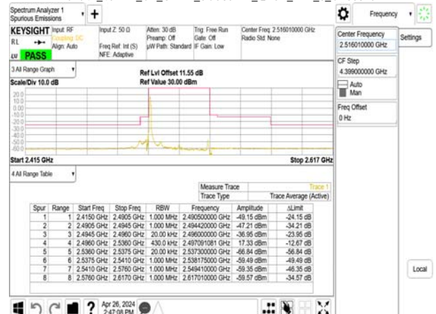
Band41_40MHz_CP_OFDM_SCS30kHz_QPSK_RB1_0_CH503202
