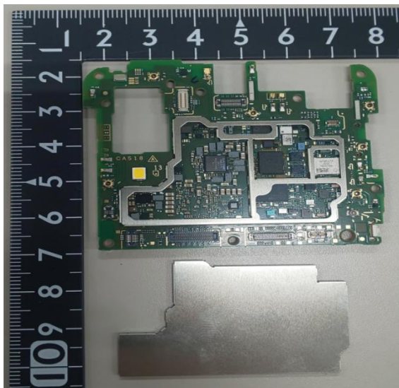
【ANT PCB】
