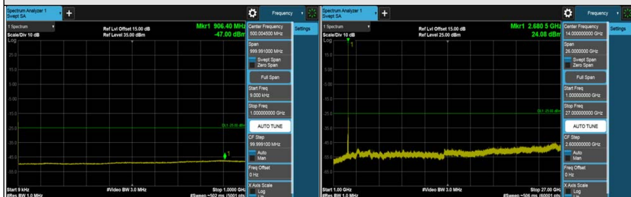
CH 41540 (2685MHz)
