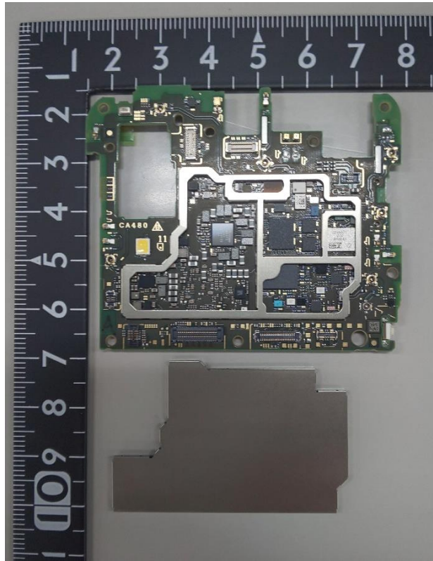
【BB PCB】
