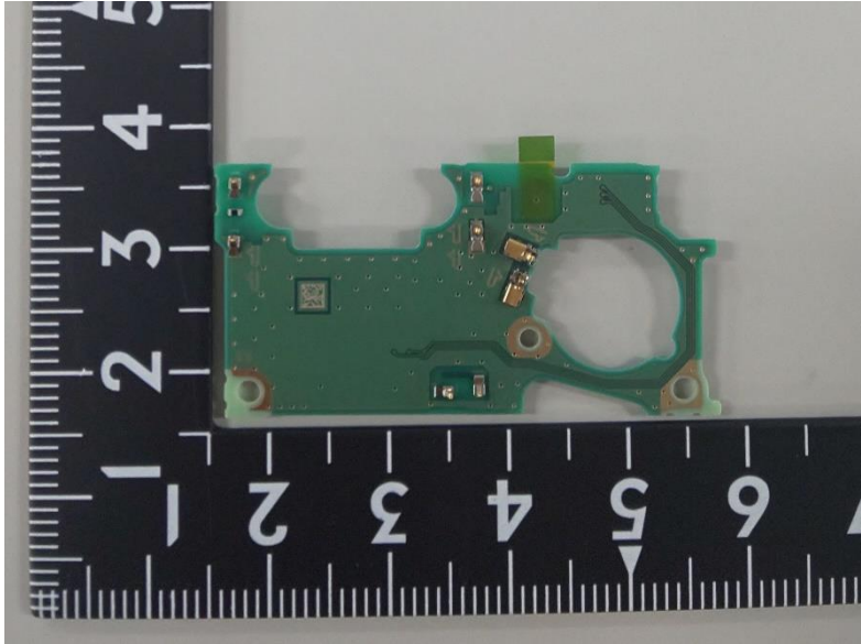
【ANT PCB】
