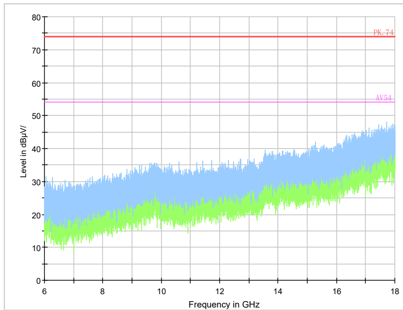
Frequency Range: 6GHz-18GHz Detector: Av mode and PK mode Modulation type: GFSK (LE 2M)
