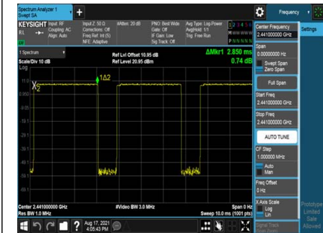
Modulation: \pi/4 DQPSK DH5 2441MHz
