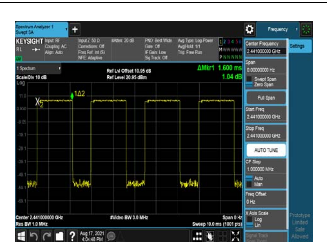
Modulation: \pi/4 DQPSK DH3 2441MHz
