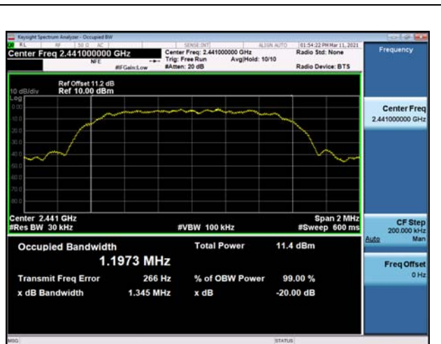
Modulation: \pi/4 DQPSK 2441MHz
