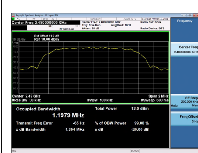
Modulation: \pi/4 DQPSK 2480MHz
