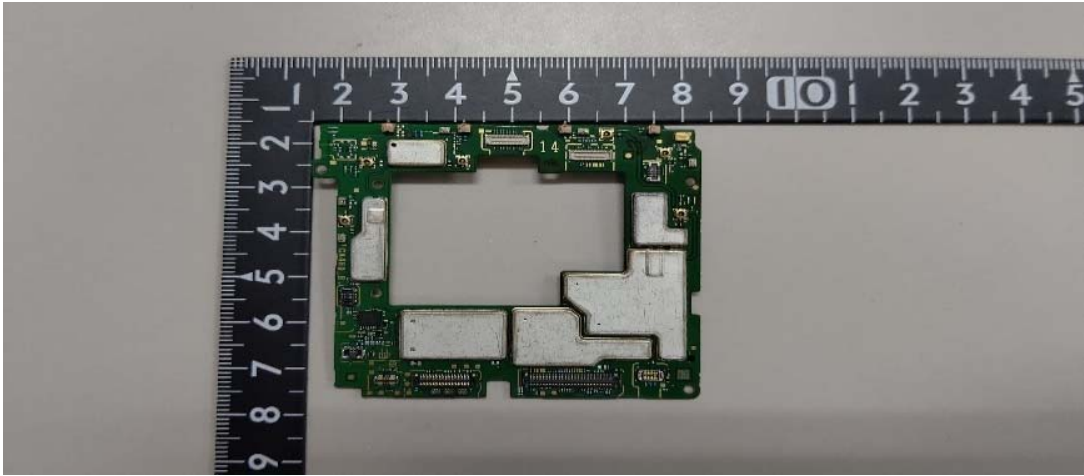
【RF PCB】
